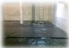
Týřovice obnova vodovodního přivaděče
