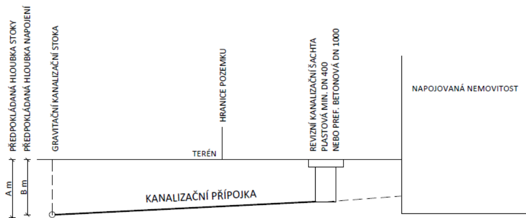
PODÉLNÉ SCHÉMA
